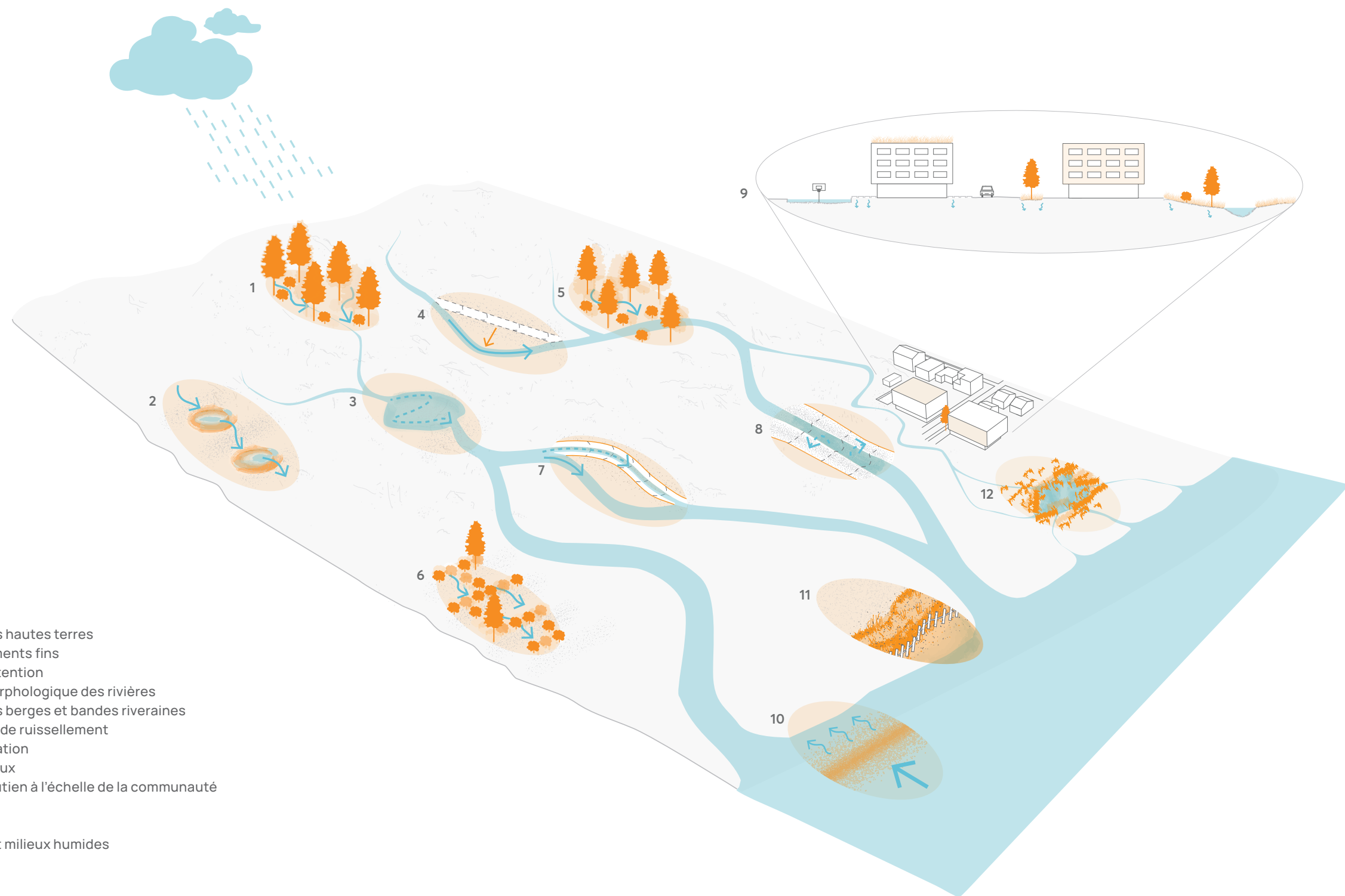
FIGURE 15 Mesures d'atténuation du risque d'inondation à l'échelle du bassin versant et des communautés © ASFQ, illustration réalisée en collaboration avec Florence Parent-Beaudin Adaptation de la figure 4.10 : Natural flood management (Barsley 2020, 87)
