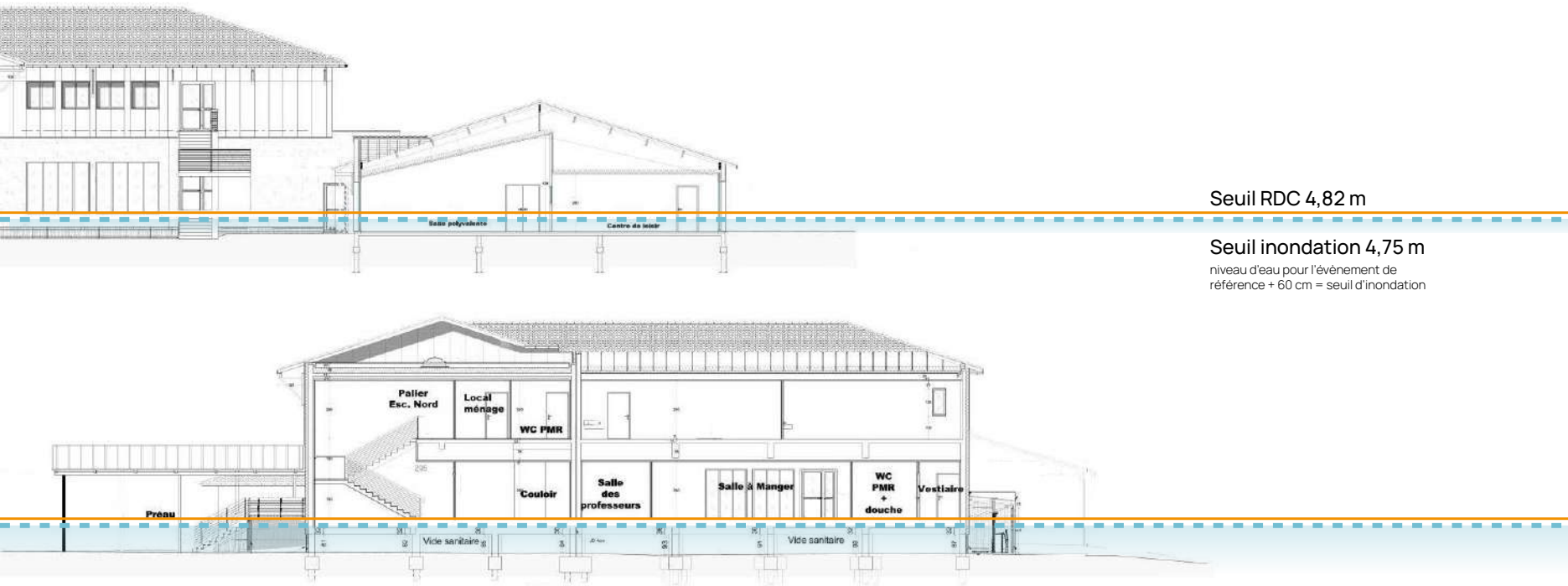
FIGURE 21 Coupes du projet, seuils de plancher et d'inondation, École Saint-Vincent-de-Paul, Bordeaux Métropole © C+M (Dessins adaptés par ASFQ)
